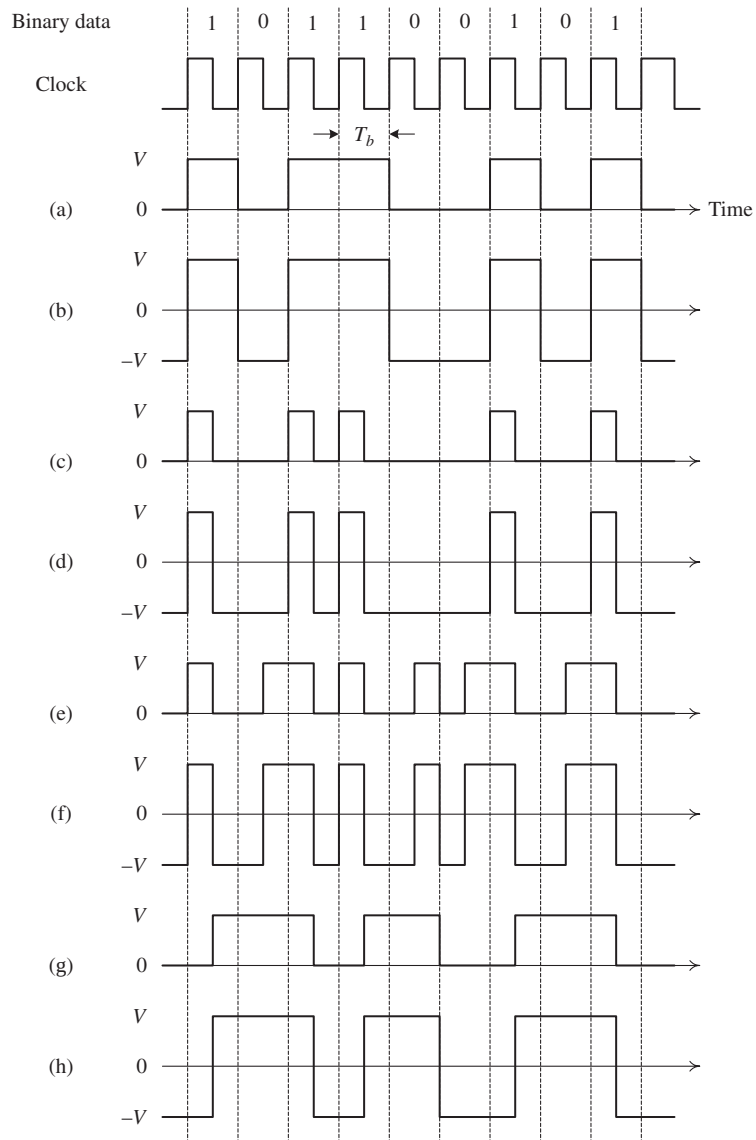
Fig. 6.1 Various binary signaling formats: (a) NRZ; (b) NRZ-L; (c) RZ; (d) RZ-L; (e) Biφ; (f) Biφ-L; (g) Miller; (h) Miller-L.
